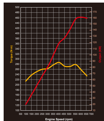
3.0-liter V6 MIVEC (Euro2 161kW/6000rpm)
